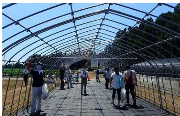
補強部材の効果や取付方法を確認する来場者
