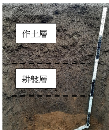
普通畑（黒ボク土）の土壌断面
