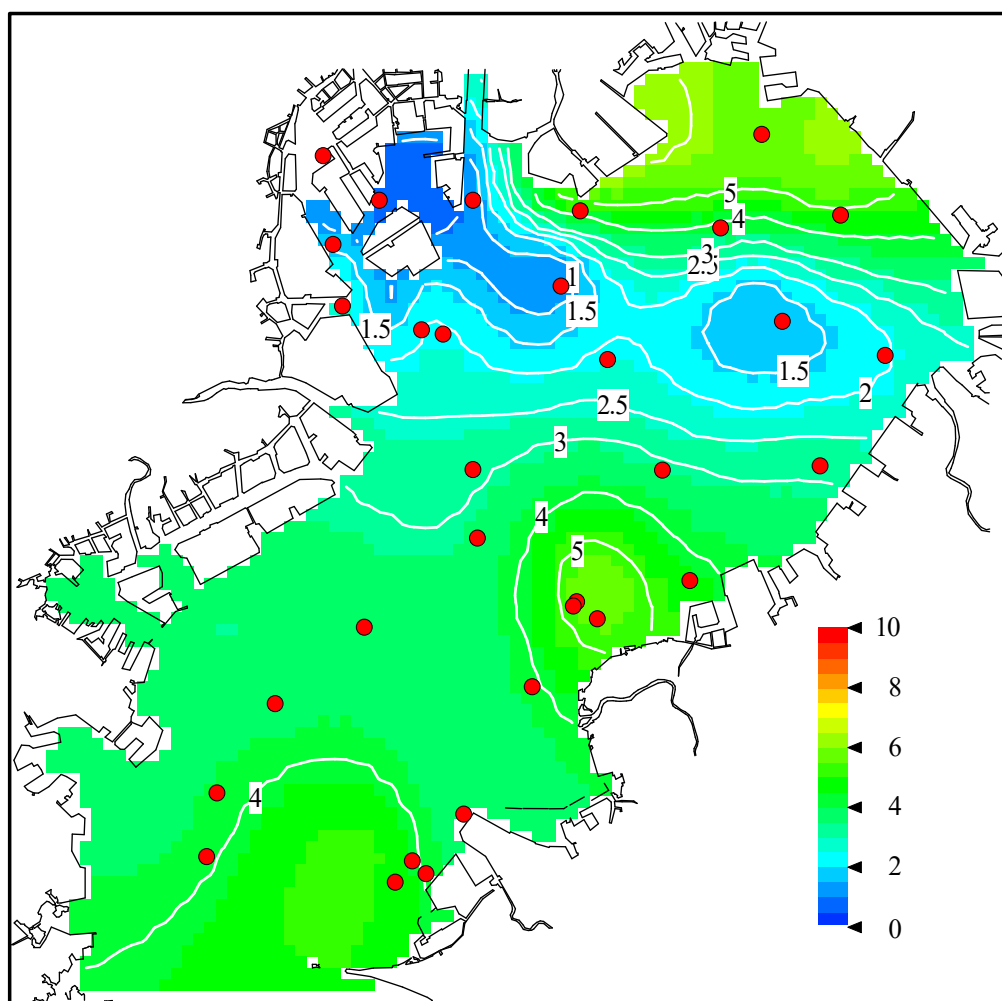
図1 底層の溶存酸素量分布
