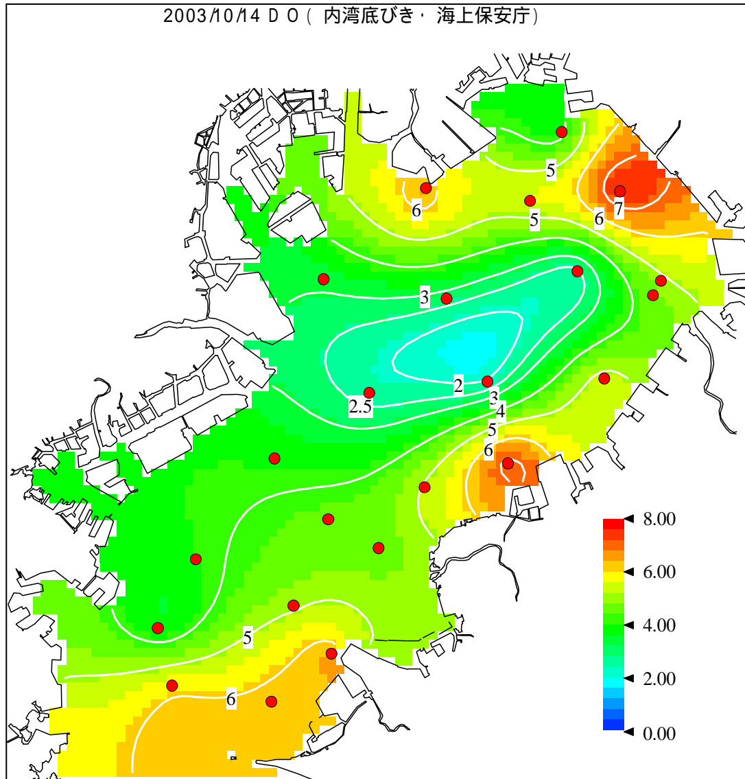
図 底層の溶存酸素量分布 (ml / L : 速報値) 平成15年10月14日観測分
