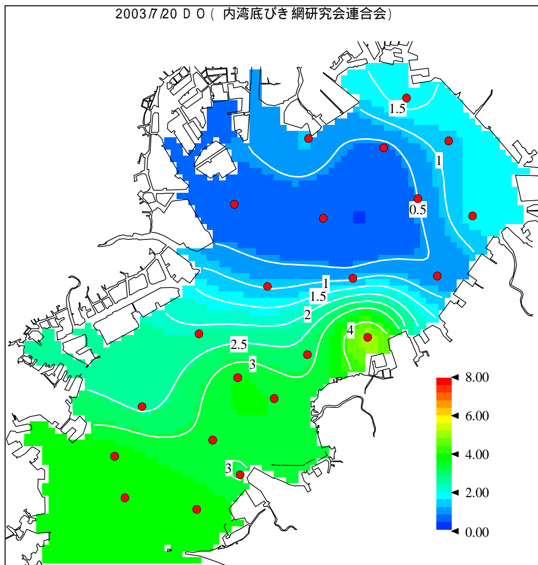
図 底層の溶存酸素量分布(ml/L:速報値) 平成15年7月20日観測分
