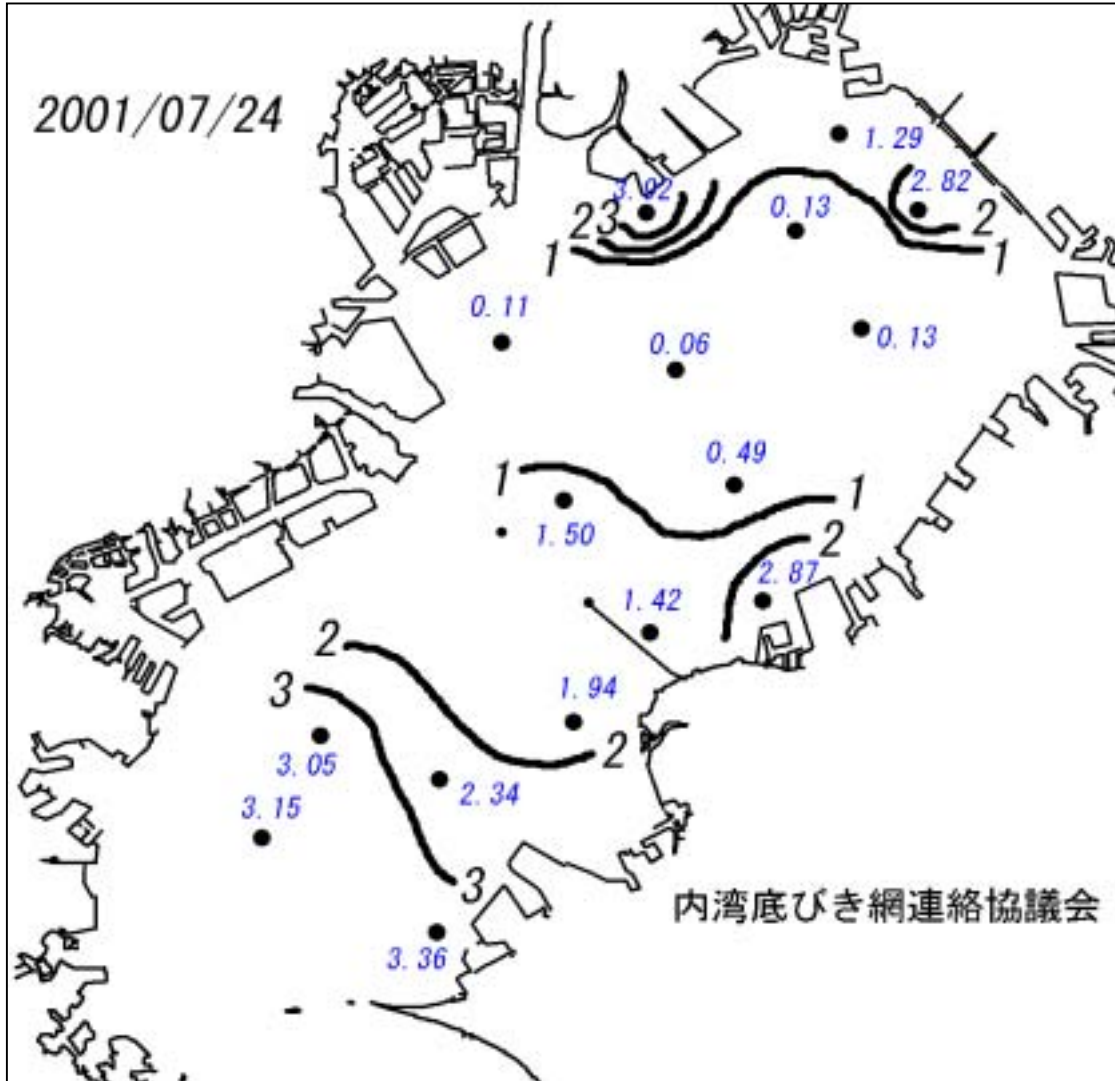
図 底層の溶存酸素量分布 (ml/L:速報値) 平成13年7月24日観測分
