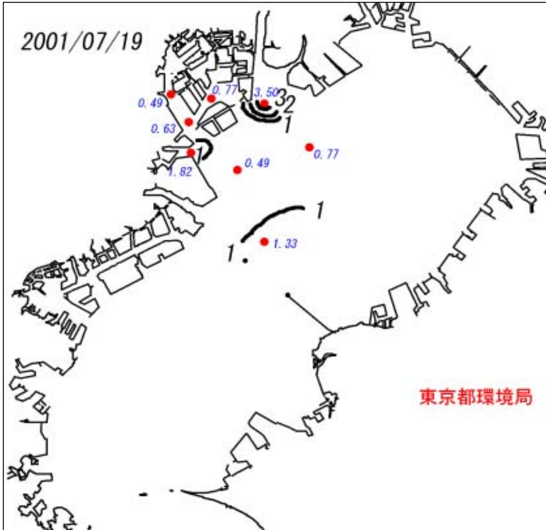
図 底層の溶存酸素量分布 (ml / L : 速報値) 平成13年7月19日観測分
