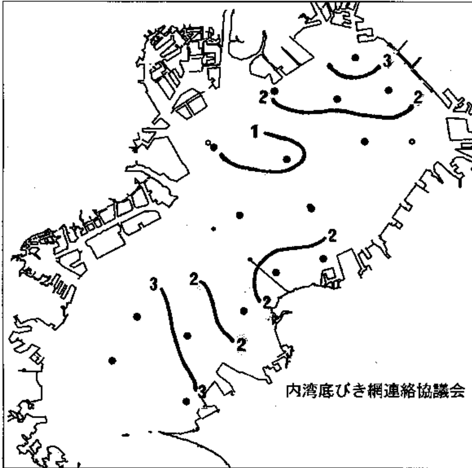
図 底層の溶存酸素量分布 (ml/L: 速報値) 平成13年6月26日観測分
