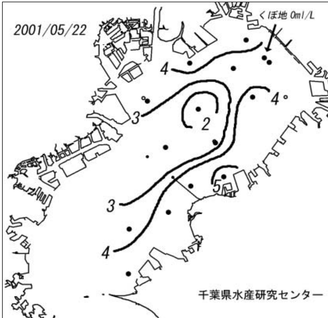
図 底層の溶存酸素量分布 (ml/L:速報値) 平成13年5月22日観測分
