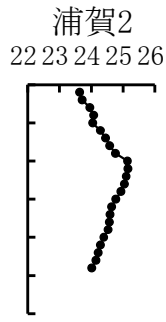
図2 縦断面の水温・塩分の鉛直分布 上：内湾，下：内房北部，右：調査ライン
