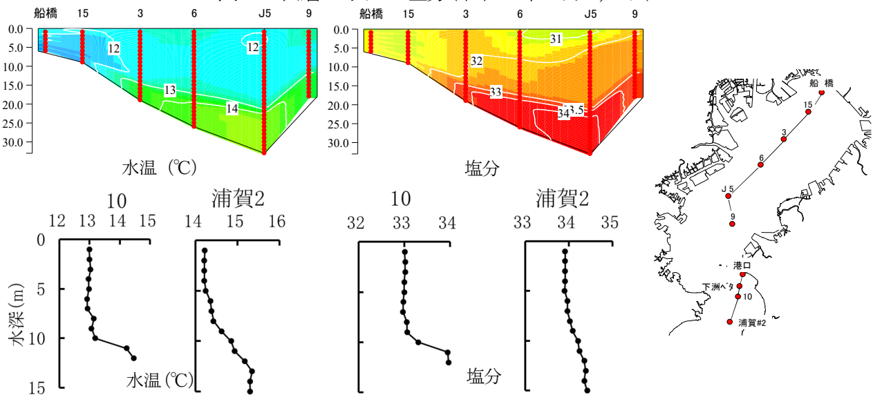
図2 縦断面の水温・塩分(令和2年3月3, 4日)
