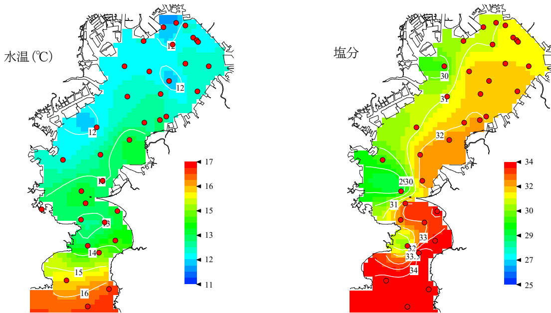
図1 表層の水温・塩分(令和2年3月3, 4日)
