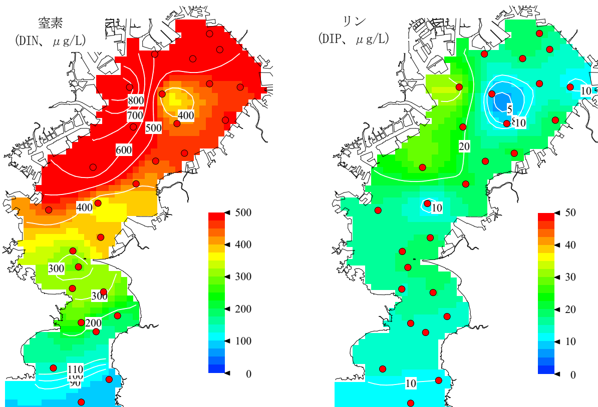
図 3 表層の栄養塩濃度の分布(令和 2 年 3 月 3, 4 日)
