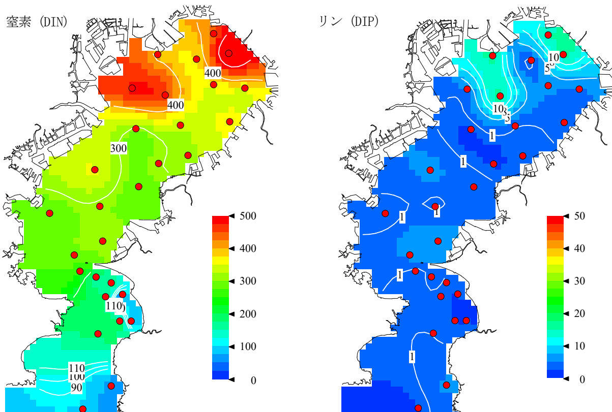
図 3 表層の栄養塩濃度 ( \mu\text{g/L} ) (平成 31 年 4 月 16, 17 日)
