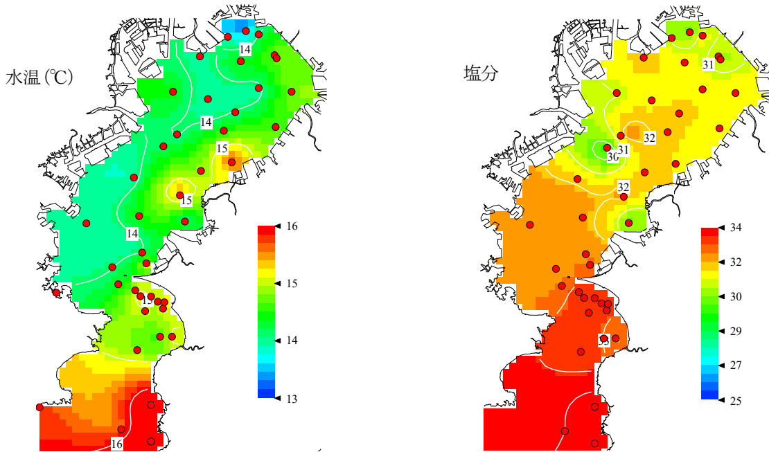
図1 表層の水温・塩分 (平成31年4月16, 17日)
