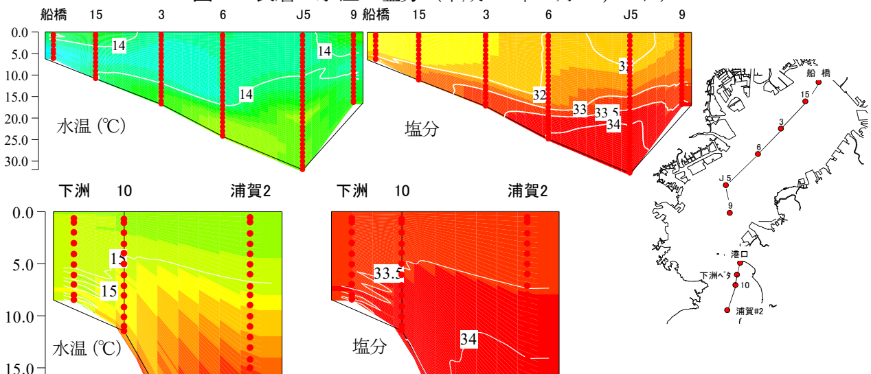
図2 縦断面の水温・塩分 (平成31年4月16, 17日)
