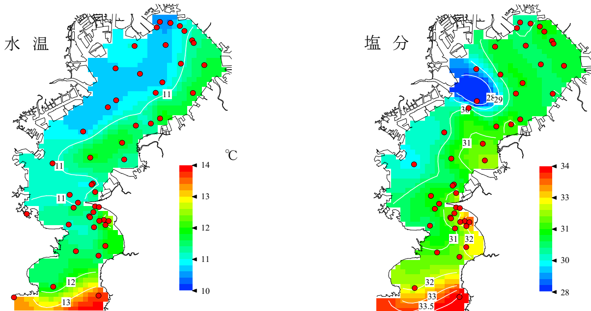
図1 表層の水温・塩分の分布(平成30年3月12日)
