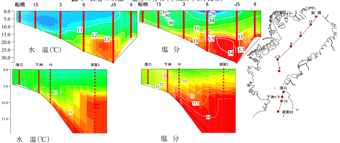
図2 調査ラインの水温・塩分の鉛直分布(平成30年3月12日) (上：内湾、下：内房北部、右：調査ライン)
