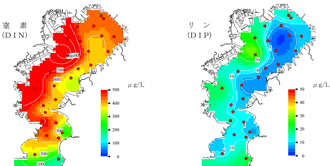
図3 表層の栄養塩濃度の分布(平成30年3月12日)
