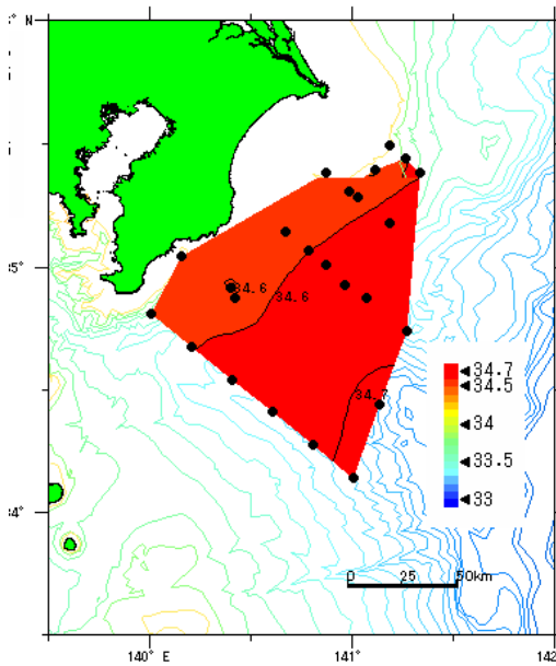
図4 水深別の塩分水平分布
