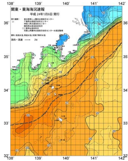
図2 関東・東海海況速報
