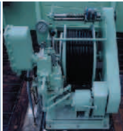
多項目水質計用ウインチ
