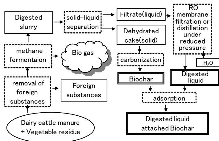
第1-2図 メタン発酵実験施設におけるメタン発酵消化液の処理フロー
