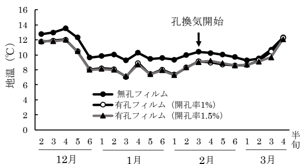
第5図 トンネル畝間マルチ栽培における換気方法別の半旬別平均地温の推移（2004～2005年）
