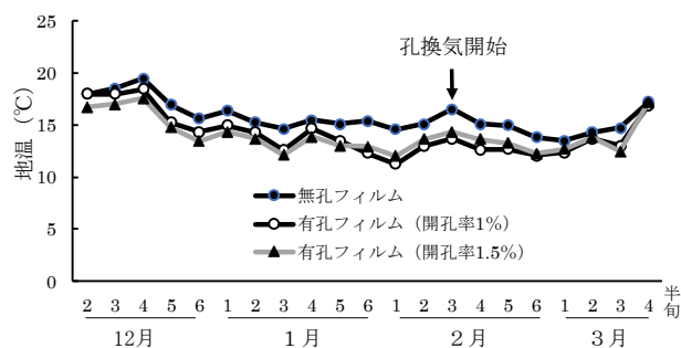
第6図 トンネル畝間マルチ栽培における換気方法別の半旬別日最高地温の推移（2004～2005年）
