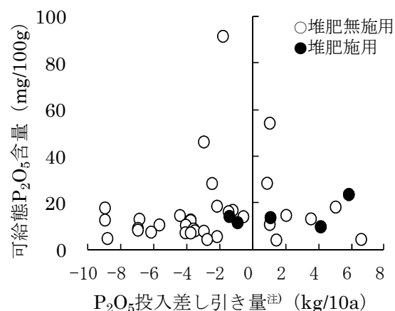
第2図 「コシヒカリ」栽培水田における P 2 O 5 投入 差し引き量と可給態 P 2 O 5 含量との関係 注) P 2 O 5 投入差し引き値 = (調査地点の肥料と堆肥の P 2 O 5 投入量の合計) - (「コシヒカリ」の P 2 O 5 施肥基準値*)
