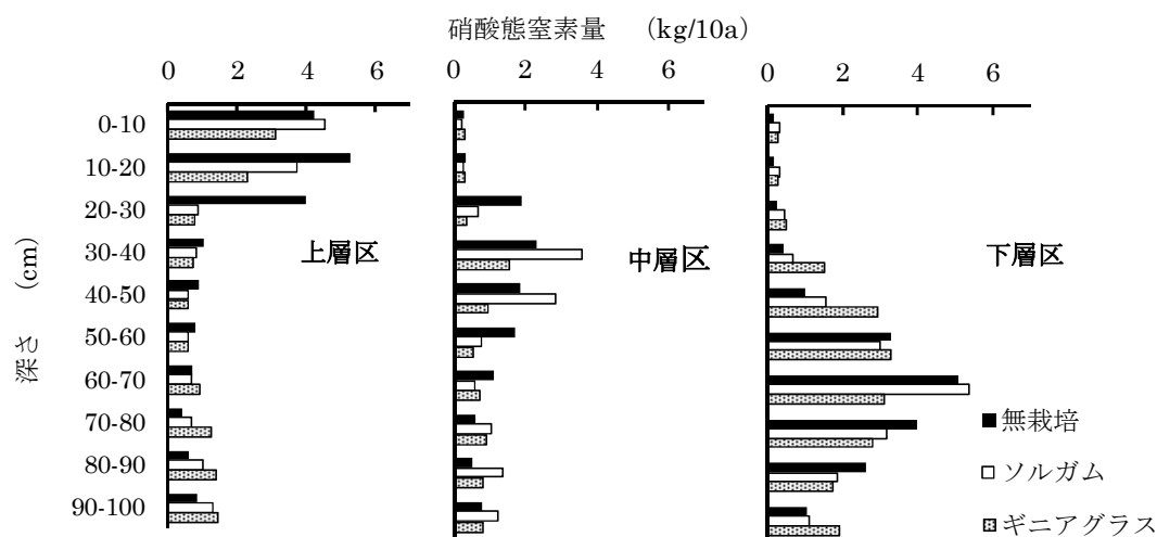
第1図 夏作緑肥作物播種前の深さ別土壤中硝酸態窒素量
