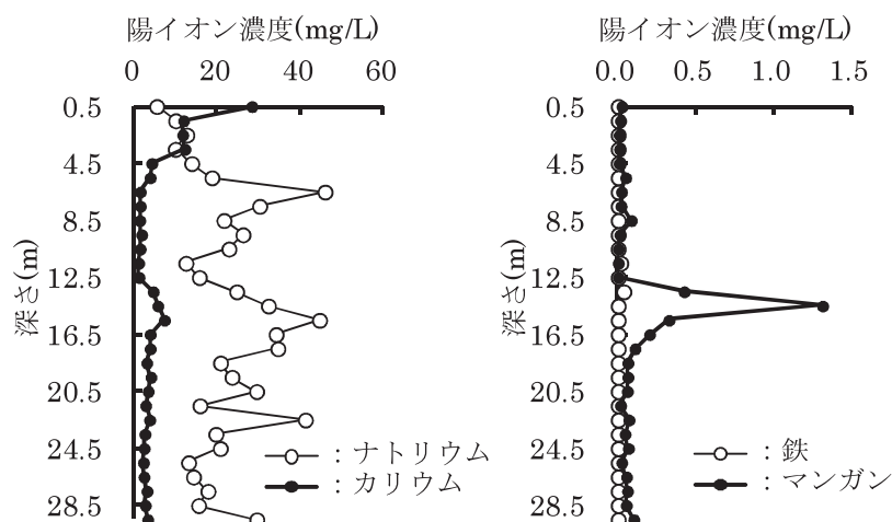
第6図 土壌水の陽イオン濃度の深さに伴う推移
