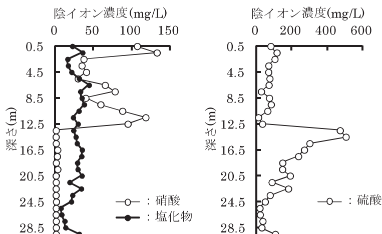
第5図 土壌水の陰イオン濃度の深さに伴う推移
