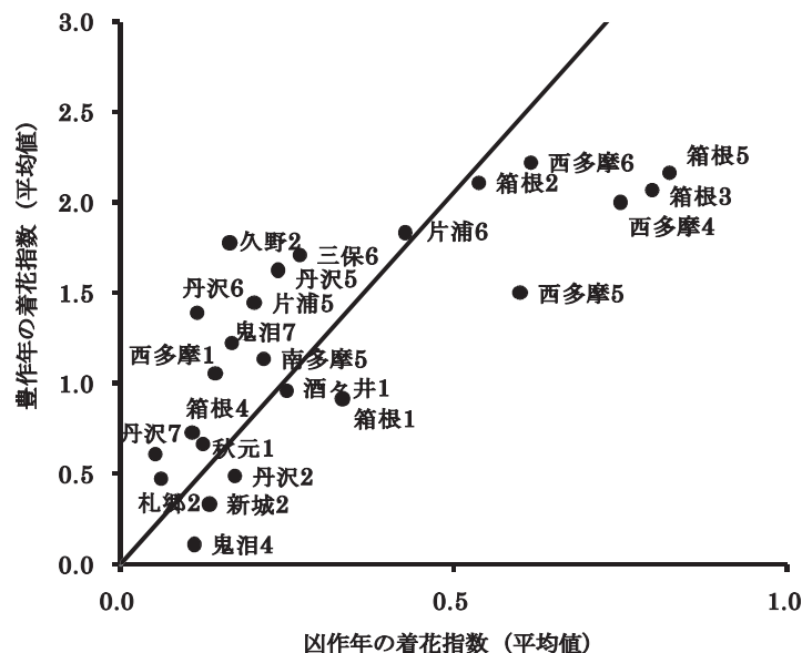
第2図 凶作年と豊作年における各クローンの平均着花指数
