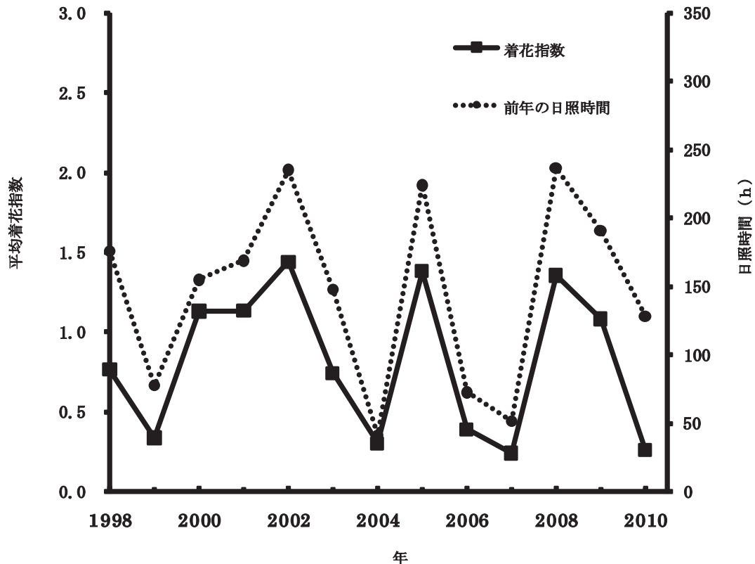
第1図 調査個体全体の平均着花指数と調査年前年の日照時間の年次変動
