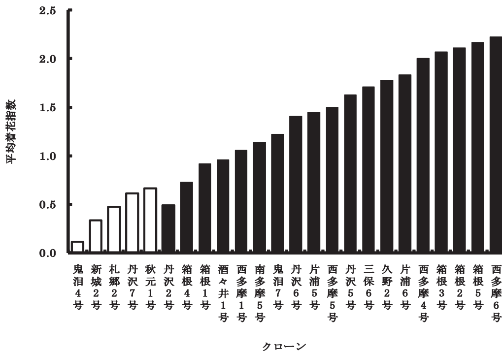
第3図 豊作年におけるクローンの平均着花指数
