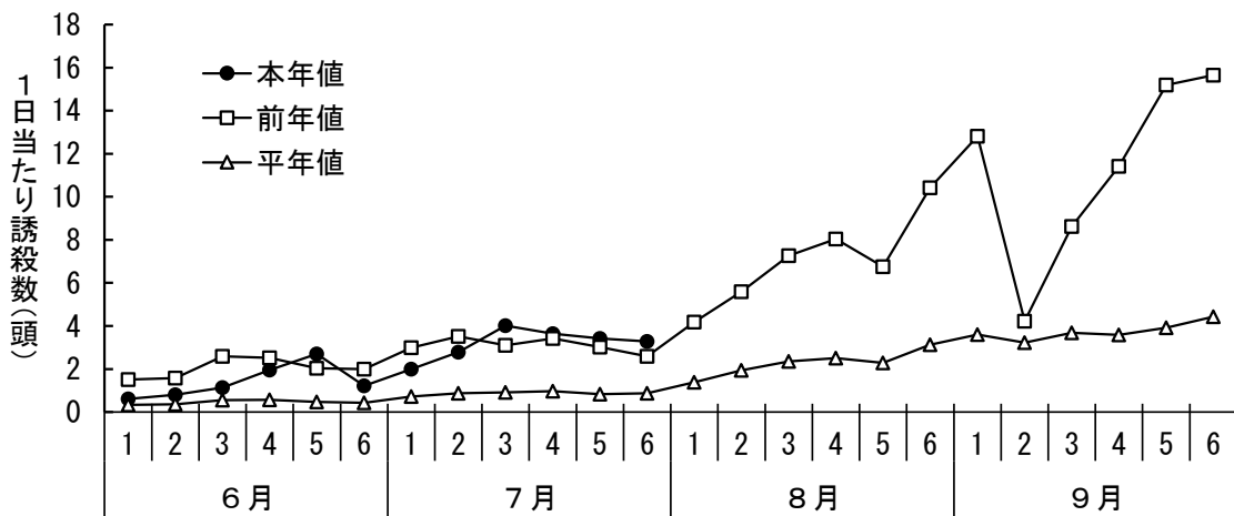
図1 フェロモントラップ調査におけるシロイチモジヨトウ誘殺数（6～9月、半旬毎）
