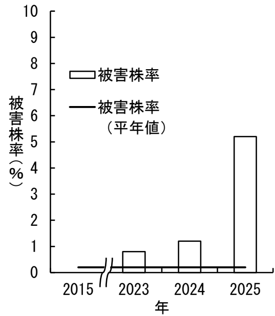
図2 8月上旬調査におけるシロイチモジヨトウ被害株率の推移
