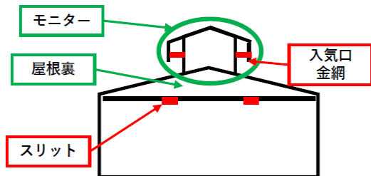
鶏舎構造(例)
