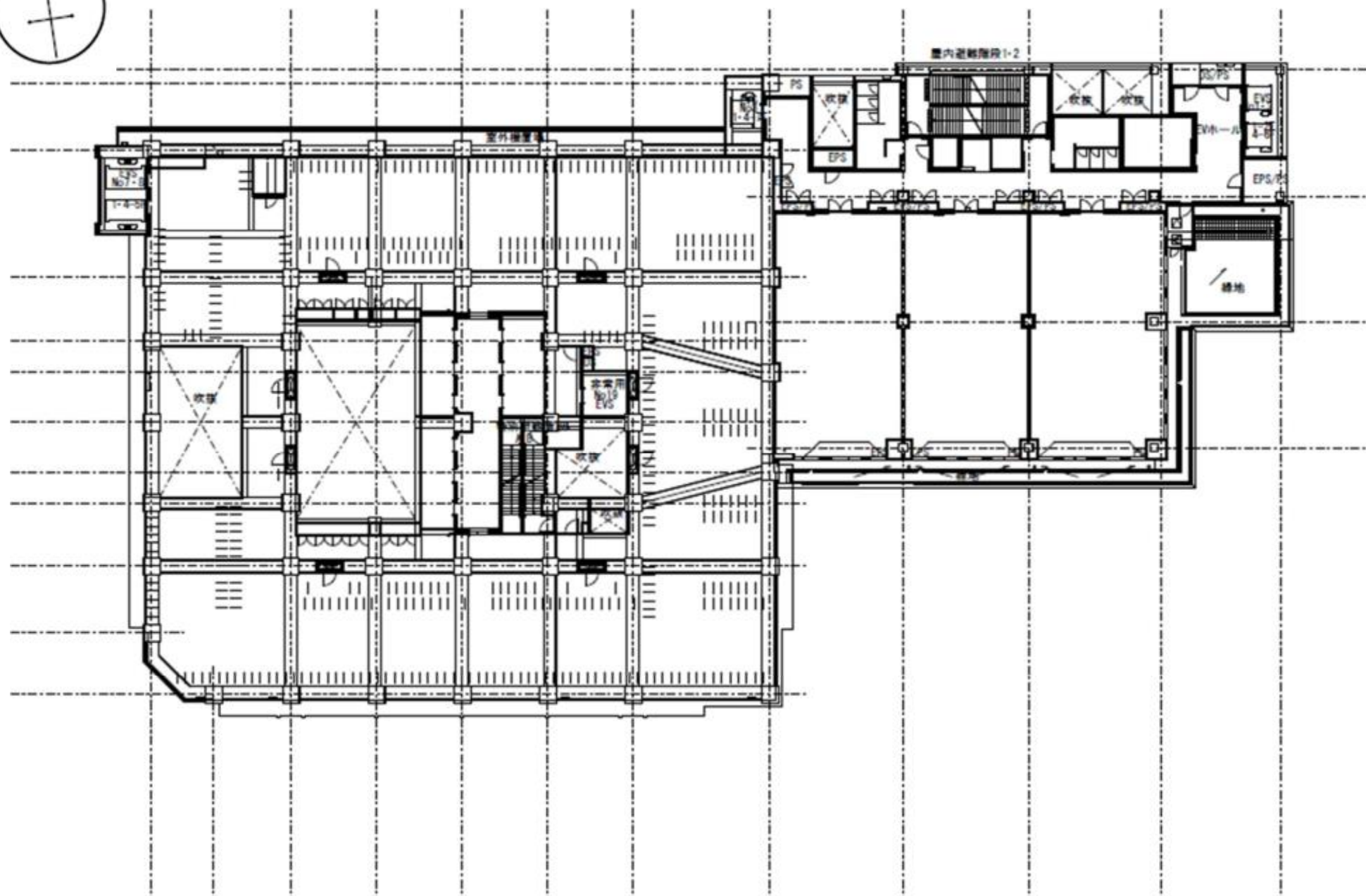
図3-6 建物配置図(5階)
