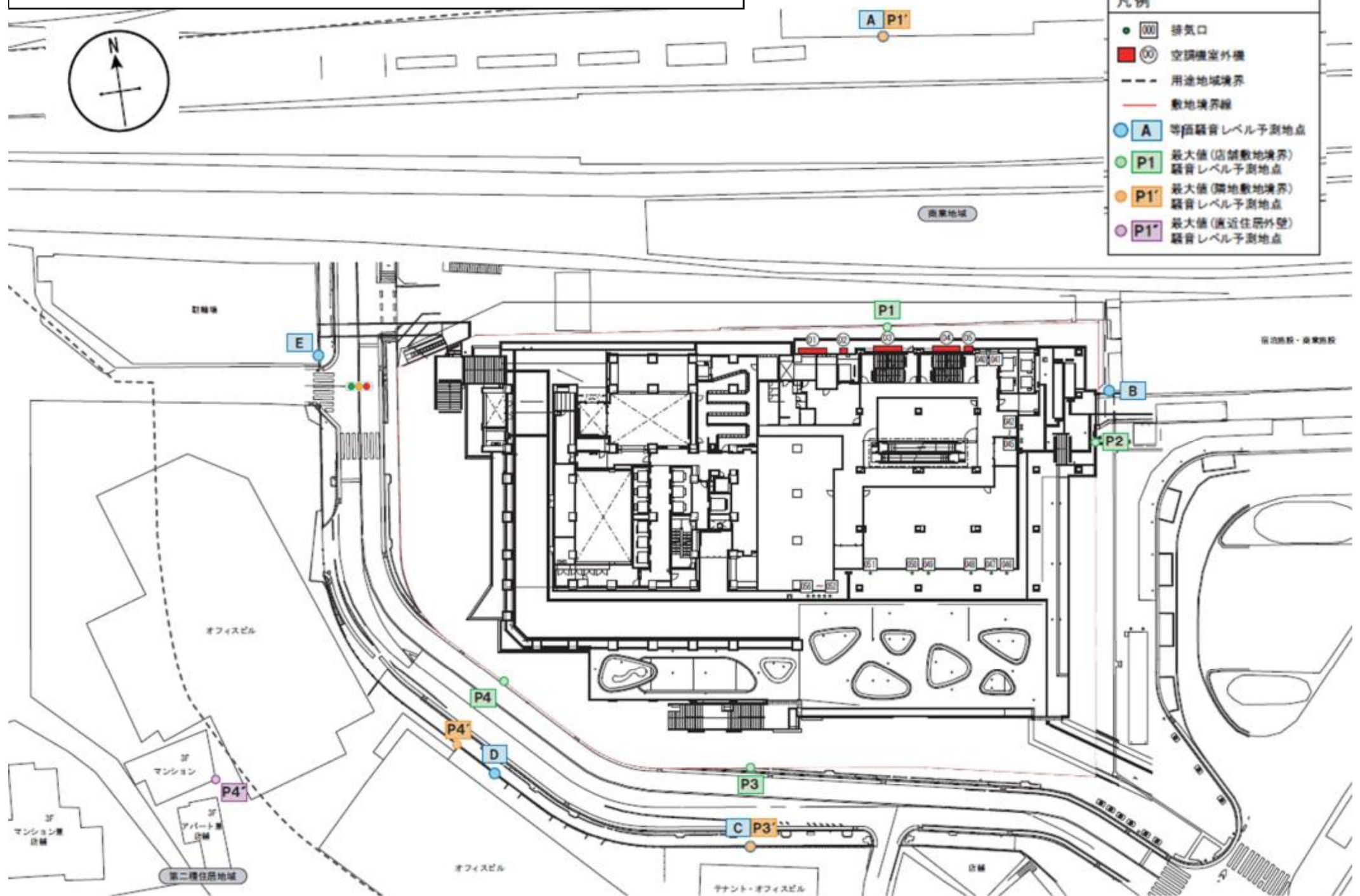
図5-2 騒音発生源及び予測地点位置図(2階)
