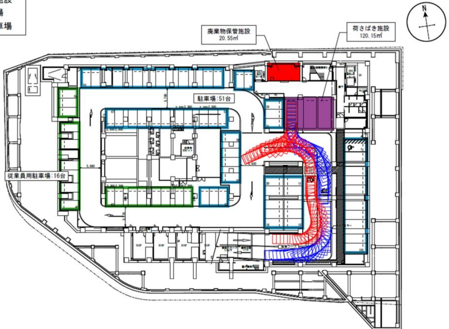
図3-2 建物配置図(地下1階)
