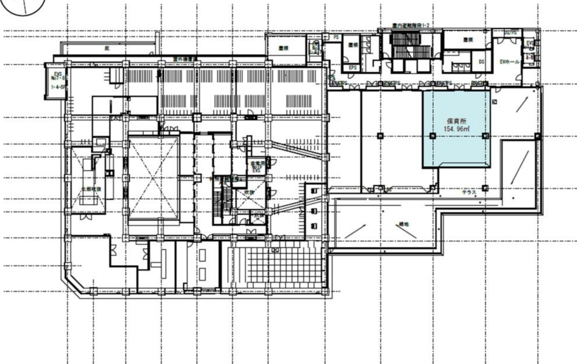
図3-5 建物配置図(4階)
