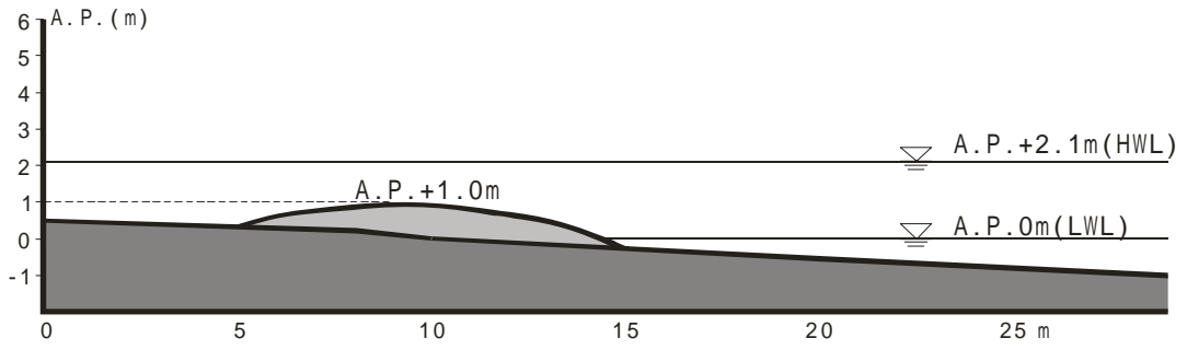
【断面】
