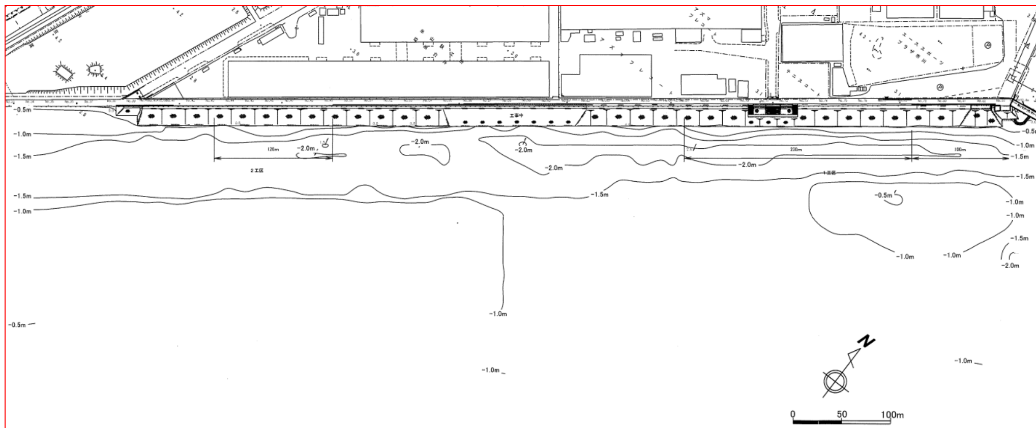
図 5-15(2) 市川市 2 丁目周辺の地盤高 (等深線図 (平成 25 年 9 月測量))
