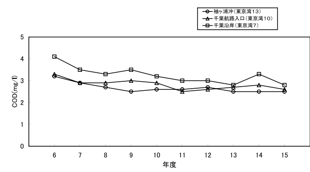
図2-10-12 海域の水質経年変化 (COD年平均値)
