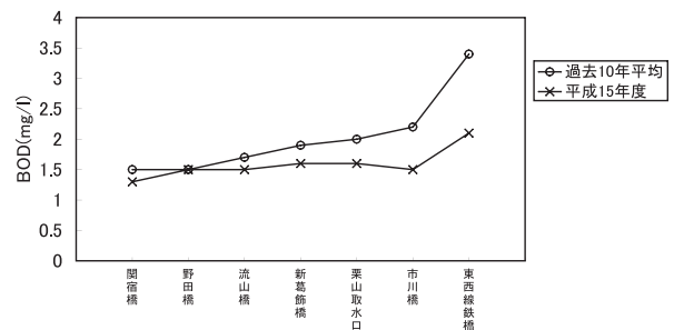
図2-10-5 江戸川の主要地点の水質経年変化 (BOD年平均値)
