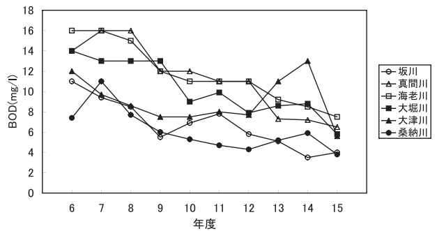
図2-10-9 県内主要河川の水質経年変化 (BOD年平均值)
