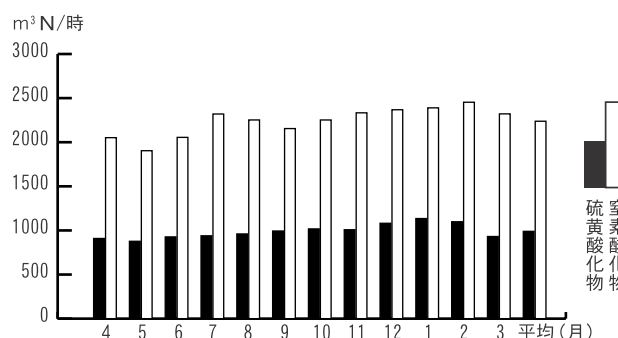
図 2-4-17 月別排出量の推移（14 年度）
