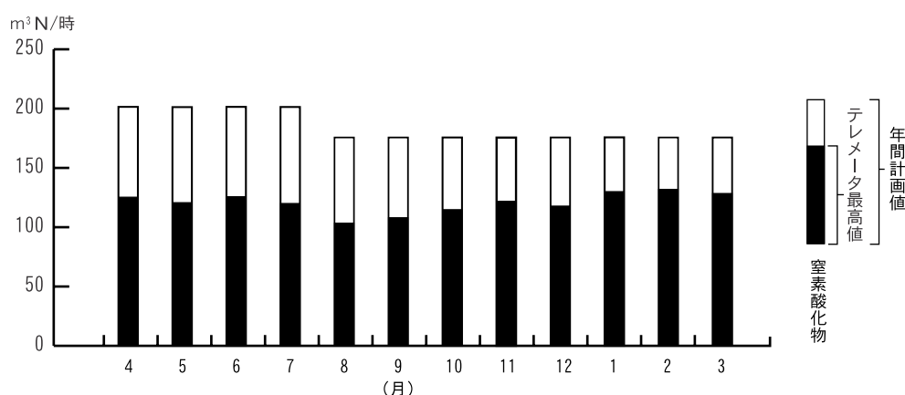
図2-4-19 年間計画値とテレメータ最高値（覚書締結4工場合計）の月別推移（14年度）
