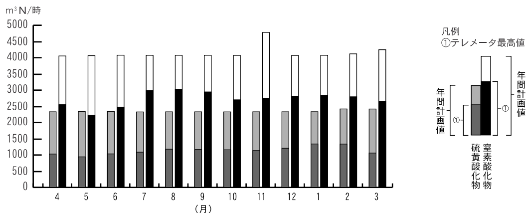
図2-4-19 年間計画値とテレメータ最高値（覚書締結4工場合計）の月別推移（14年度）
