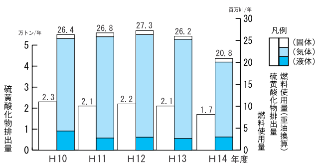
図 2-4-3 県内主要工場・事業場における硫黄酸化物排出量及び燃料使用量の経年変化
