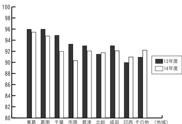
図2-4-8 光化学オキシダント環境基準の時間達成率の地域別平均値（13～14年度）
