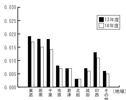
図 2-4-7 一酸化窒素の地域別年平均値（13～14年度）
