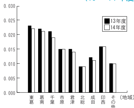
図 2-4-7 一酸化窒素の地域別年平均値（13～14年度）
