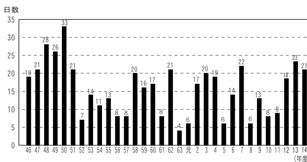
図2-4-10 光化学スモッグ注意報発令日数の年度別推移
