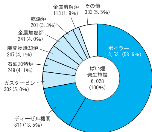
図 2-4-1 ばい煙発生施設の種類の状況 (千葉県を除く 15 年 3 月末現在)
