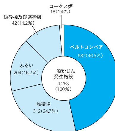
図 2-4-2 一般粉じん発生施設の種別別状況 (12年3月末現在)
