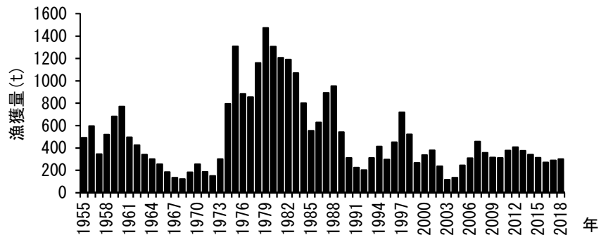
サザエ漁獲量の経年変化 (千葉農林水産統計年報, 漁業・養殖業生産統計)
