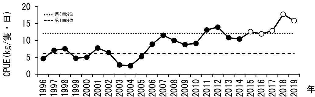
サザエ主要地区刺網漁業 CPUE の経年変化
