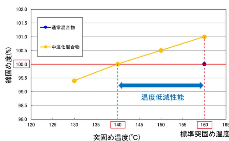
図2-6 温度—突固め度のグラフ（作成例）
