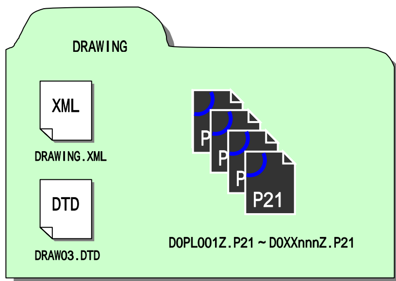
図 6-10 図面フォルダ (DRAWING) の格納イメージ
