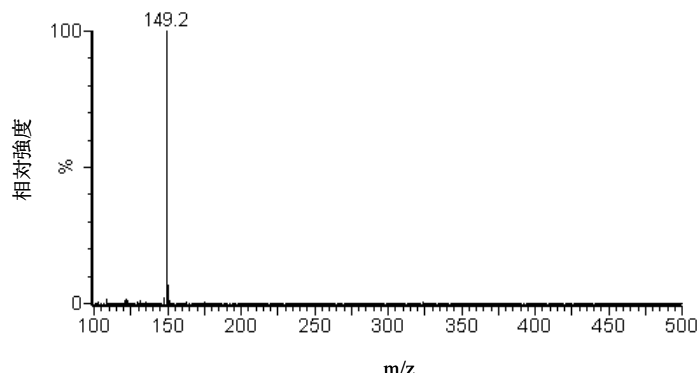
図3 製品3 未知成分のマスペクトル (LC/MS ESI ネガティブモード コーン電圧: 40V)
