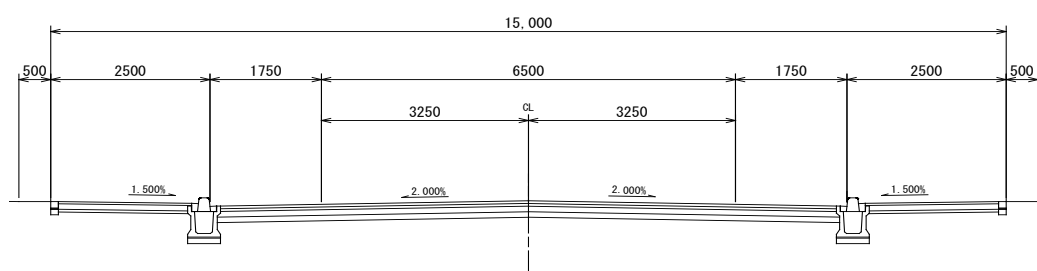
標準断面図
