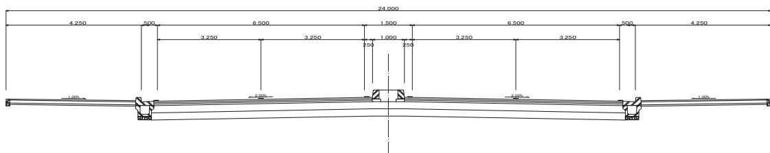
《標準断面図》
