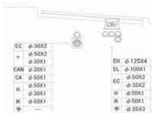
《標準断面図》
