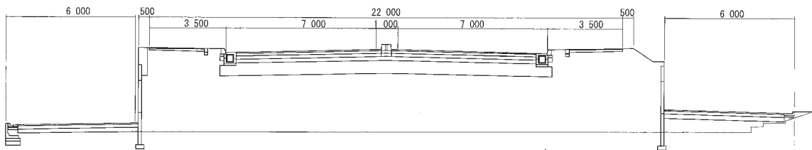
橋梁部
