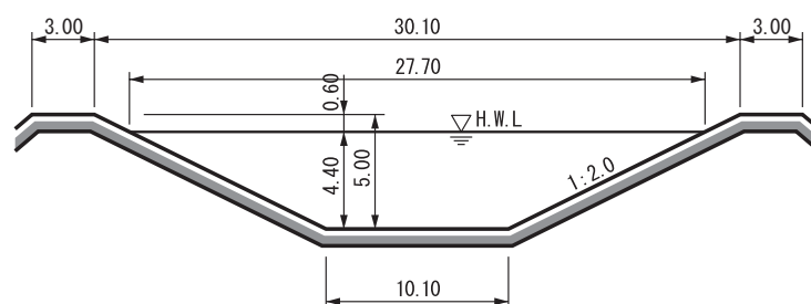
《代表断面図》(加曾利町地先 大宮橋上流)
