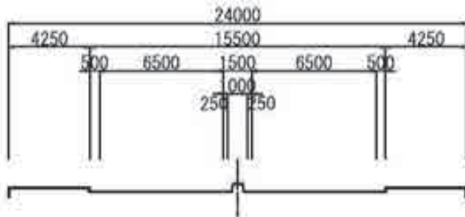
一般部
