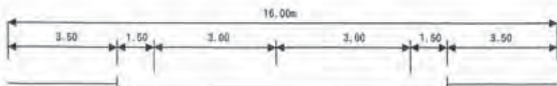
《標準断面図》
