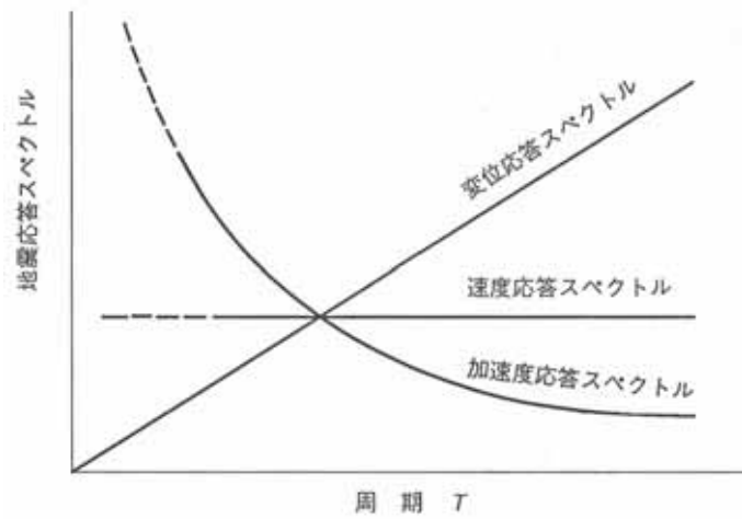
図 4.4-4(2) 地震応答スペクトルの概略の形
