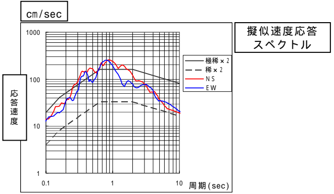
図 4.4-6(1) 既存波形と地震応答スペクトル
