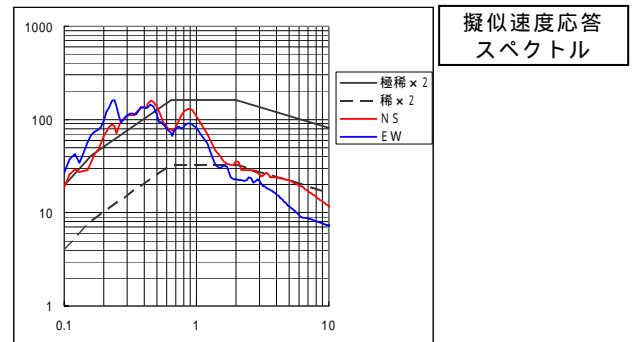
図 4.4-6(2) 既存波形と地震応答スペクトル
