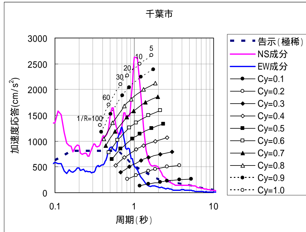
図 4.4-7 ハイブリッド合成後の地表における速度波形および 5%加速度応答スペクトル，性能等価応答スペクトル（千葉）
