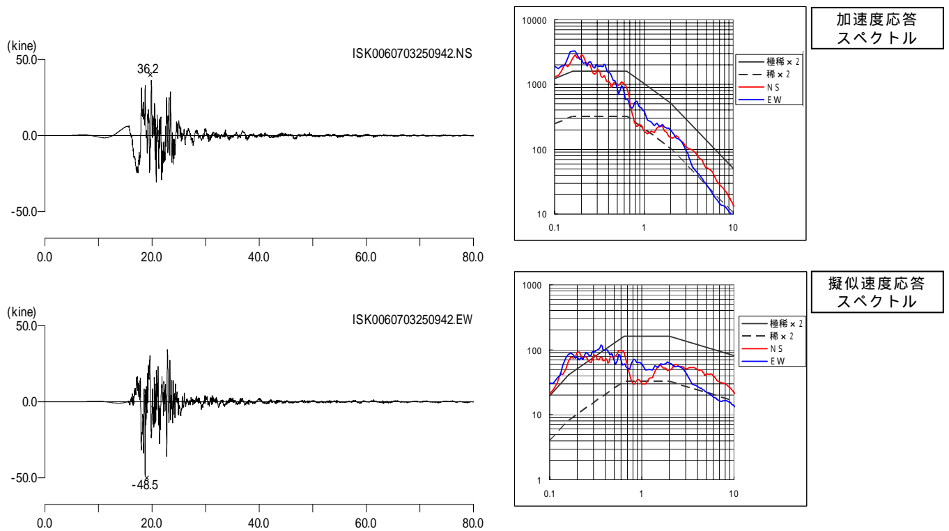
図 4.4-6(3) 既存波形と地震応答スペクトル 2007年能登半島沖地震 K - N E T ISK006 富来
