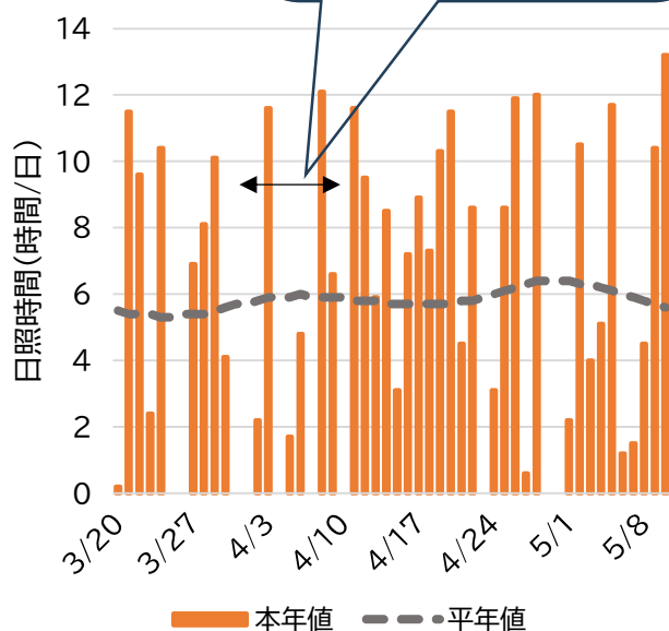
図2 日照時間の推移(アメダス、横芝光)
